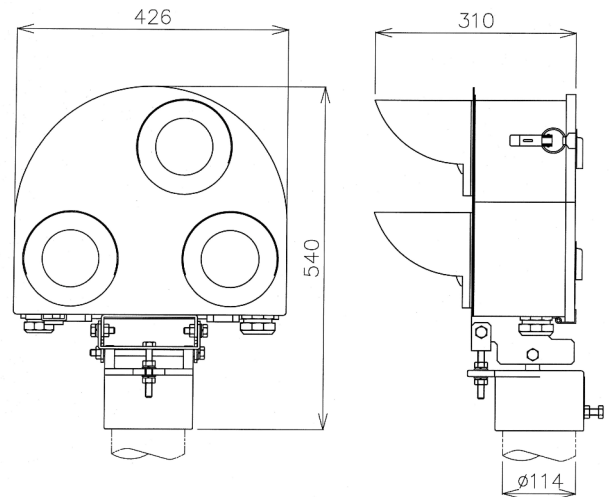
【外観図】
