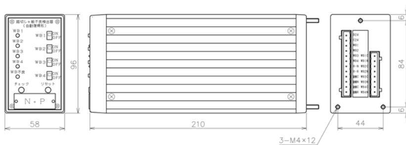
【外観図】
