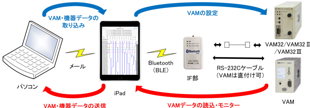
【構成図】
