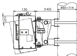
【外観図】
