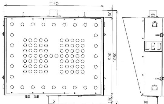
【外観図】
